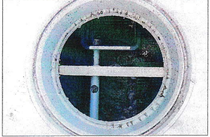
写真2 一次処理装置の内部状況
